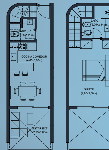
PLANTA - DUPLEX 1 + 1 1/2
